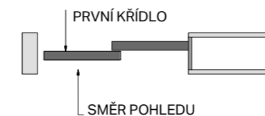
Stavební pouzdro NORMA PARALLEL – pravě
