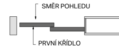
Stavební pouzdro NORMA PARALLEL – levě
