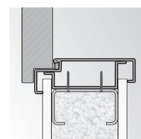
rohová zárubeň velká montáž na sádkartónovou stěnu
