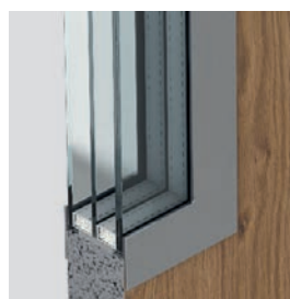
Prosklení – trojskelná sada třídy P4
