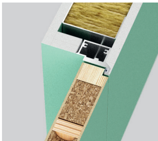
Reverzní polodrážka (otevřené dovnitř) - levé dveře
