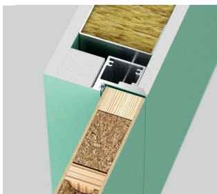
Bezpoldrážkové standard (otevřené ven) - pravé dveře
