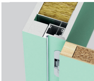
Bezpoldrážkové standard (otevřené ven) - pravé dveře
