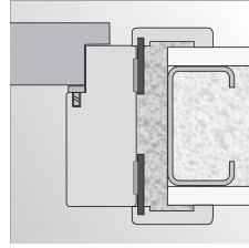
montáž na pěnu do sádkartónové
