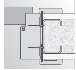
montáž na vruty do stěny ze sádkartónu
