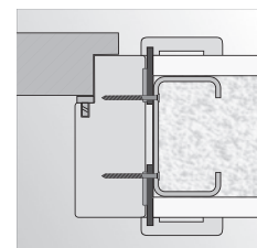
montáž na vruty do stěny ze sádkartonu
