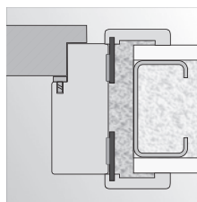
montáž na pěnu do stěny ze sádkartonu
